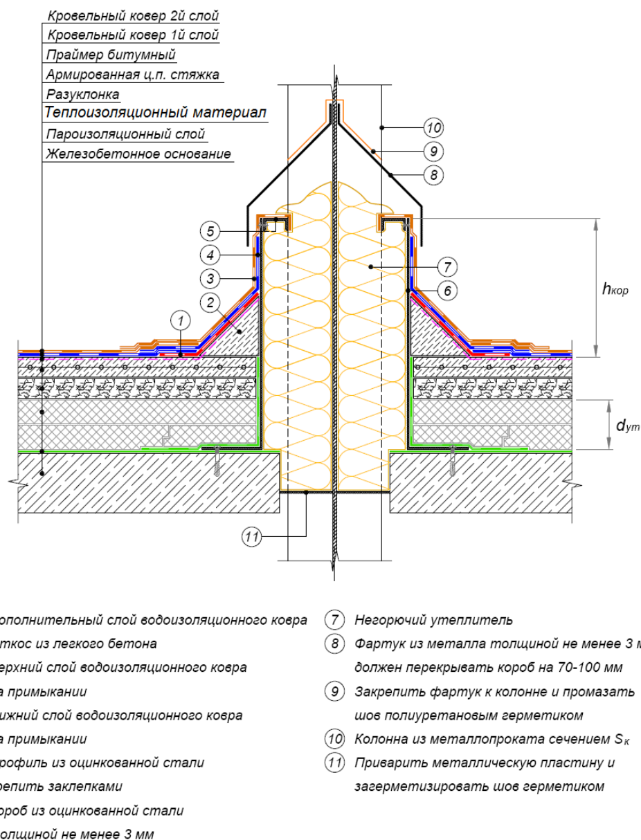
Рисунок Г.13 – Схема прохождения колонны через совмещенное кровельное покрытие Вариант 2
