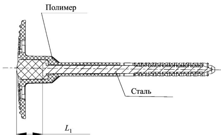
Рисунок Г.2 – Схема тарельчатого анкера
